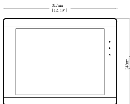
正视图
