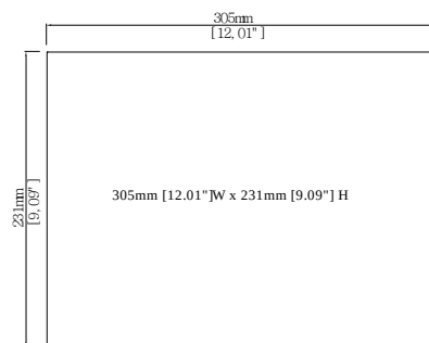
开孔尺寸图
