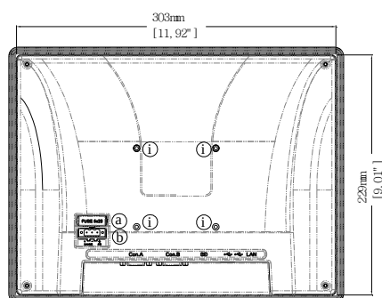
背视图
